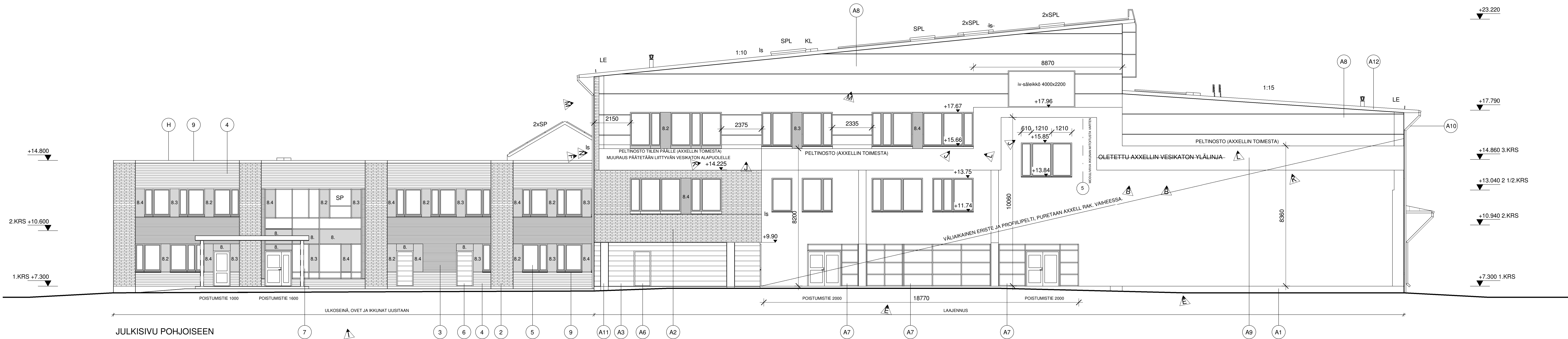
JULKISIVU POHJOISEEN
